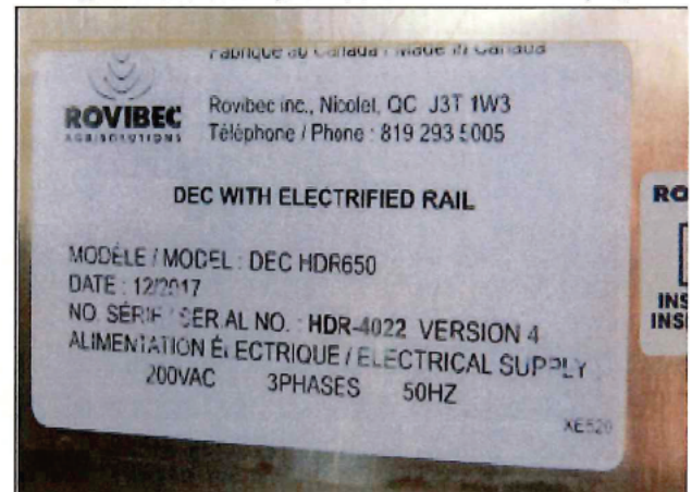
【自動給餌機（製造番号：HDR-4022）】
